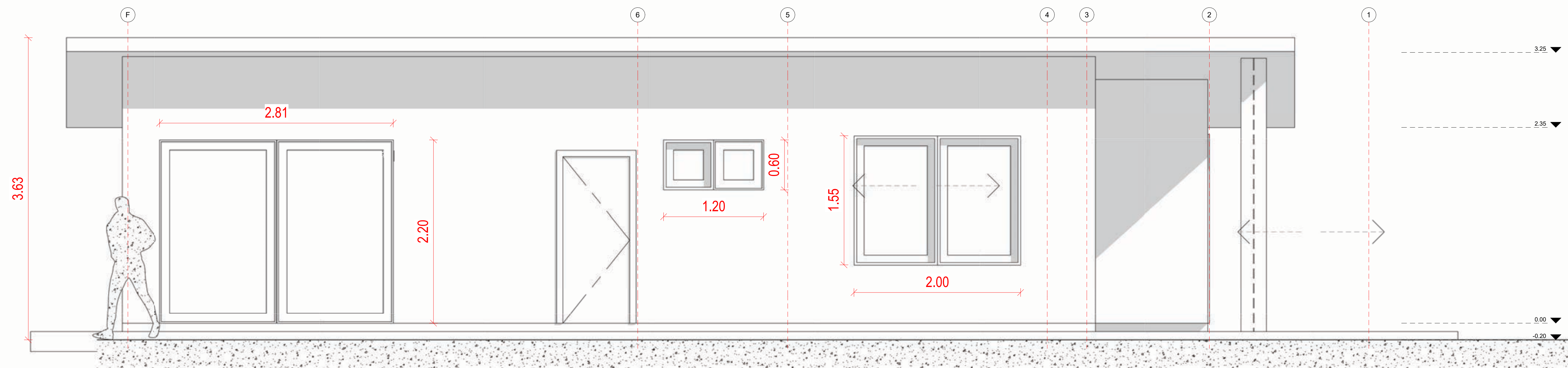
Norte Copia 1 1 : 25
