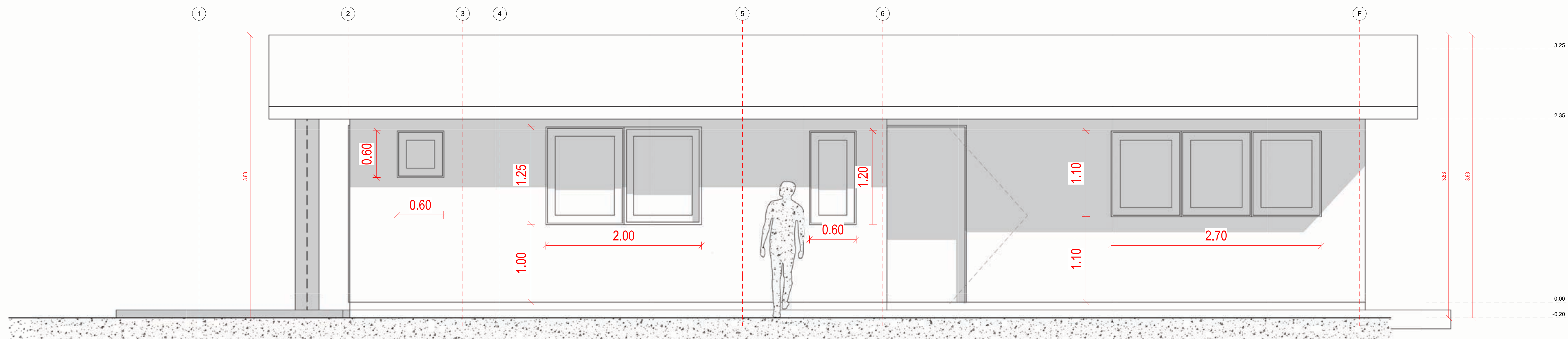
Sur Copia 1 1 : 25
