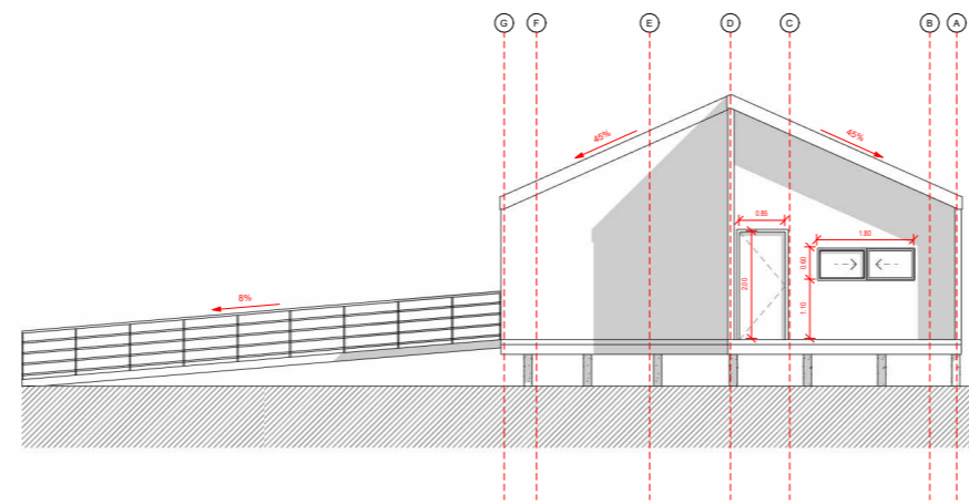
Alzado Norte 1 : 50
