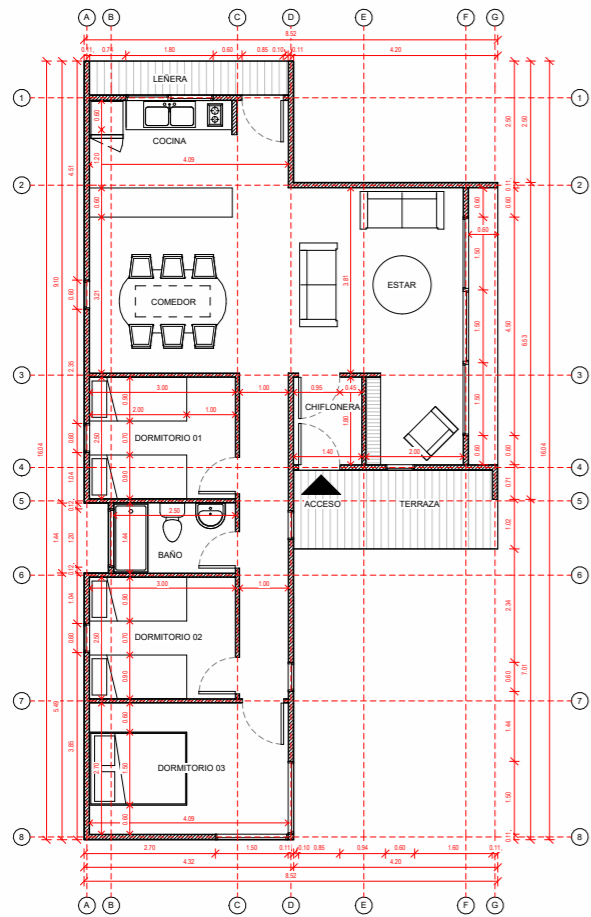
Planta Primer Nivel 1 : 50
