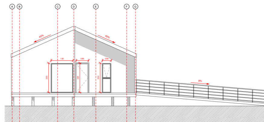
Alzado Sur 1 : 50
