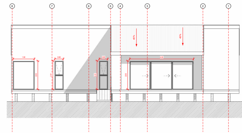
Alzado Oriente 1 : 50
