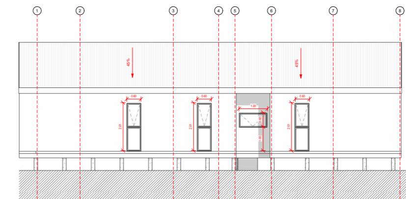
Alzado Poniente 1 : 50
