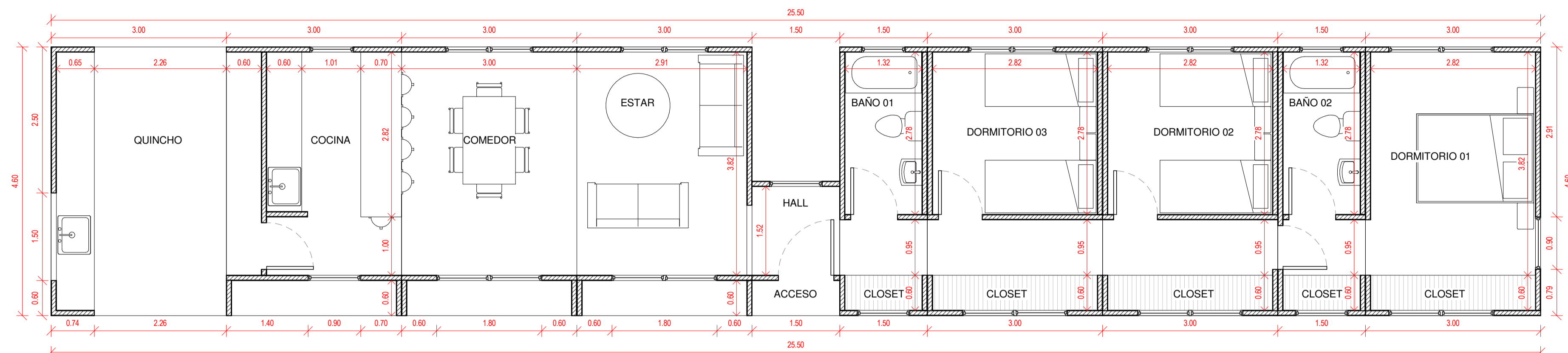
Planta Primer Nivel 1 : 50
