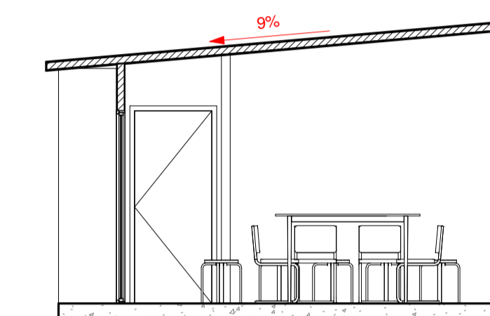
Sección 1 1 : 50
