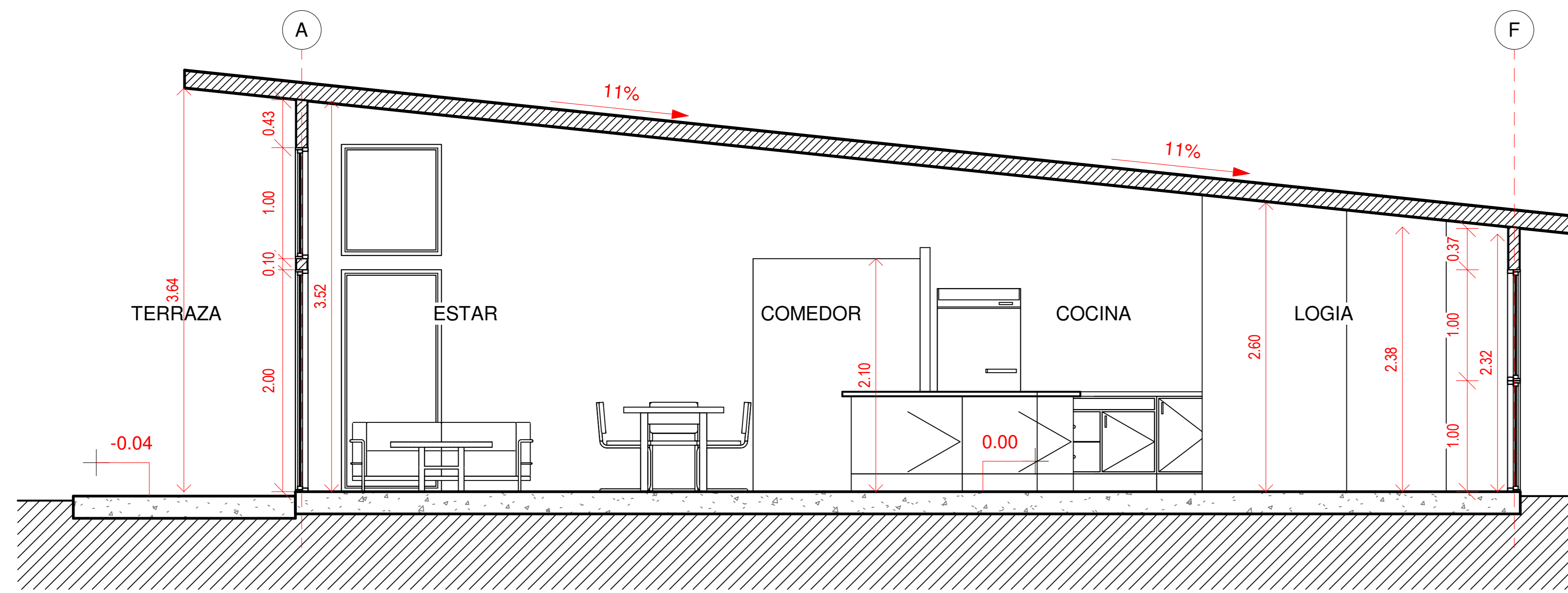
Sección A-A' 1 : 50
