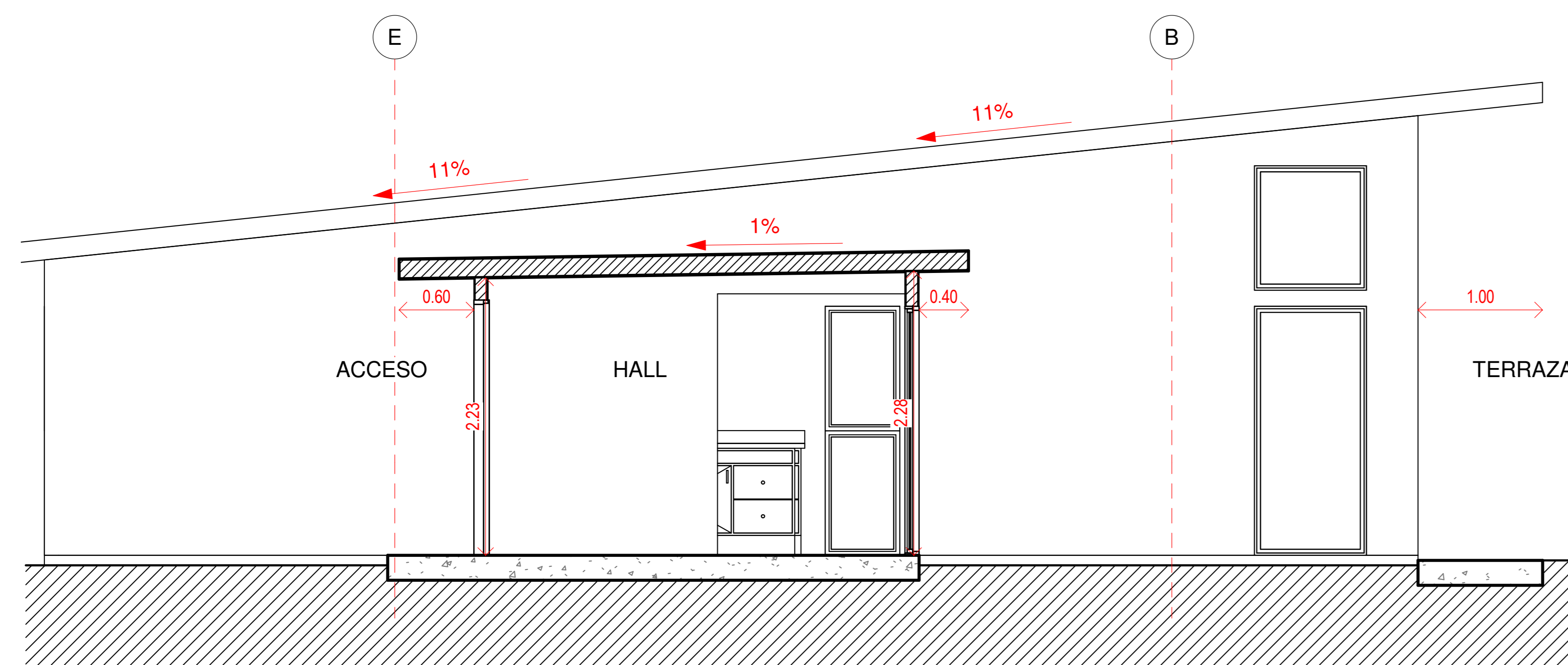
Sección C-C' 1 : 50
