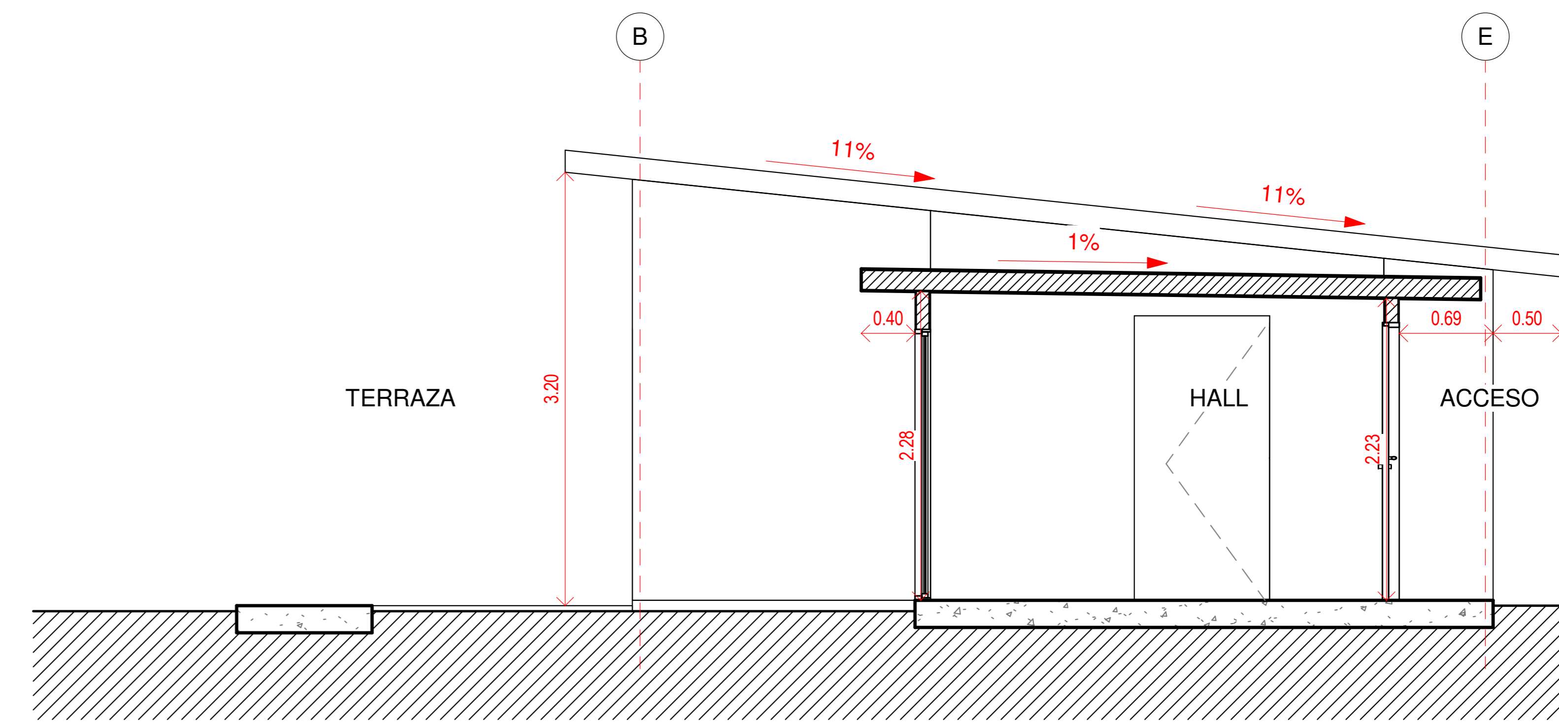
Sección B-B' 1 : 50
