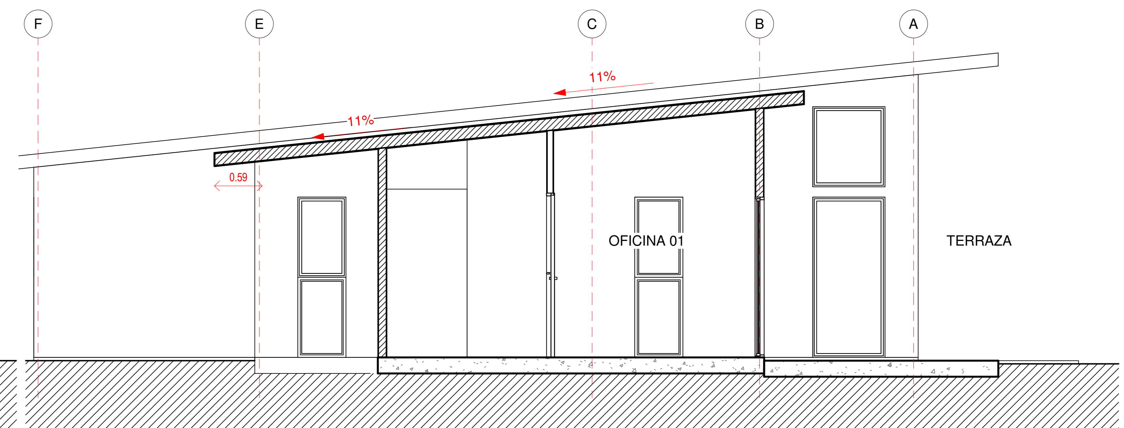
Sección D-D' 1 : 50
